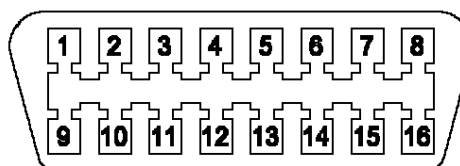
Pinbelegung des Diagnosesteckers am Fahrzeug, Vorderansicht
