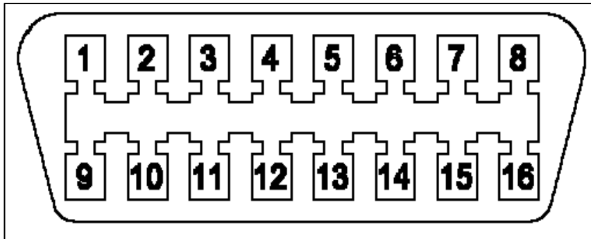
OBD Buchse
