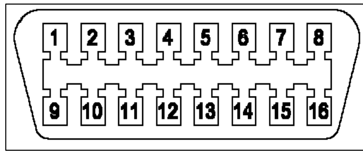
OBD Buchse
